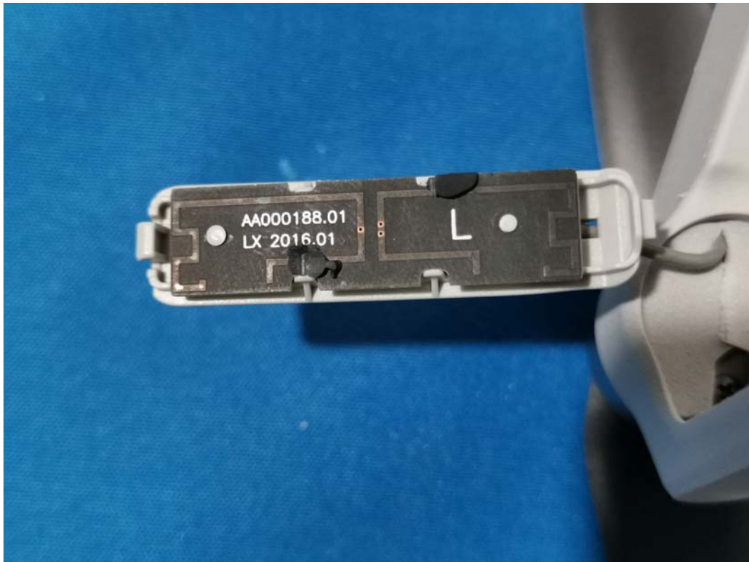
Antenna Chain 1(SDR/WIFI&BLE)
